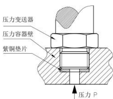
螺纹前端面密封安装图
