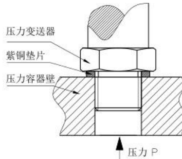
六角端面密封安装图
