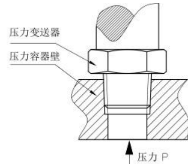
锥度螺纹密封安装图
